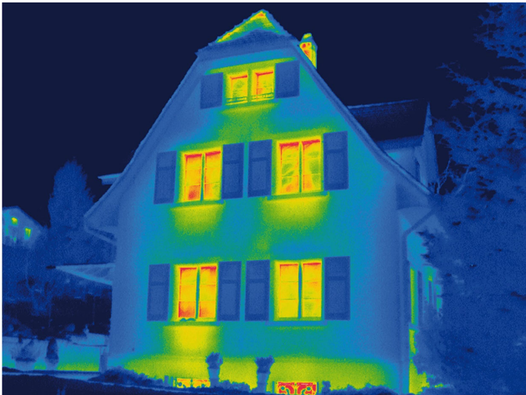
Wärmebildaufnahme eines Wohnhauses: Die gelb-roten Bereiche zeigen deutlich, wo Wärme über Fenster und Fassaden entweicht.
