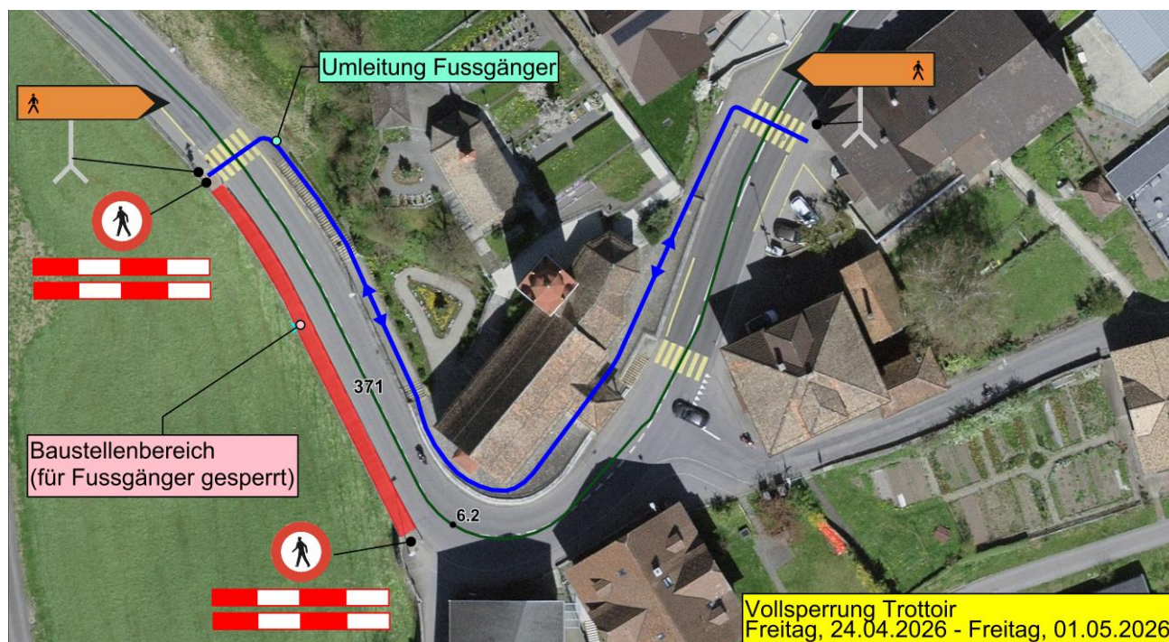
Abbildung 1: Luftbild Trottoirauskragung Chilerank, Steinerberg. Baustellenbereich (rote Fläche) und Umleitung Fussgängerverkehr (blaue Linie).
